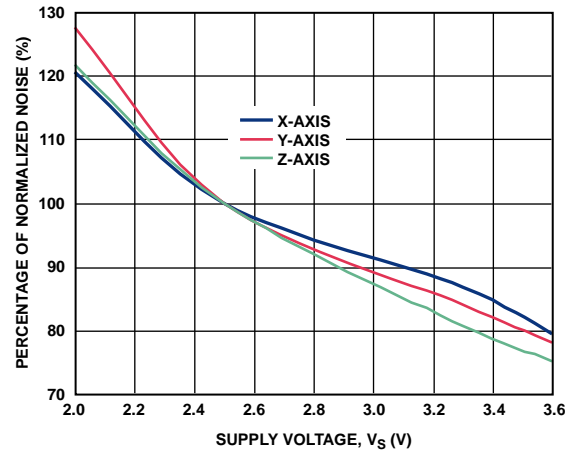
图52. 归一化的噪声与电源电压 V_s
