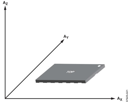
图56.加速度灵敏度轴(沿敏感轴加速时相应输出电压增加)
